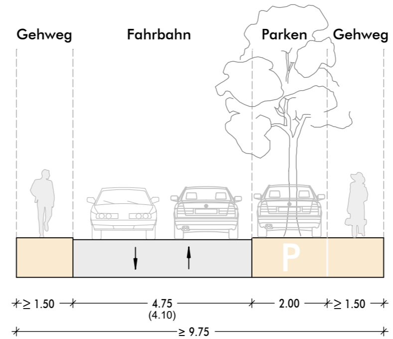
D - Straßenraum mit einseitigem Gehwegparken
