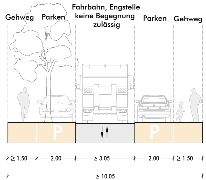
C - Straßenraum mit beidseitigem Gehwegparken
